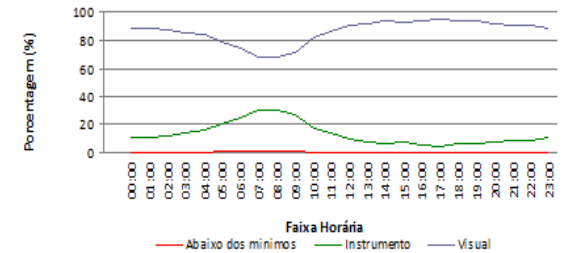
Operacionalidade em porcentagem (Teto 100 ft e visibilidade de 400 m)
