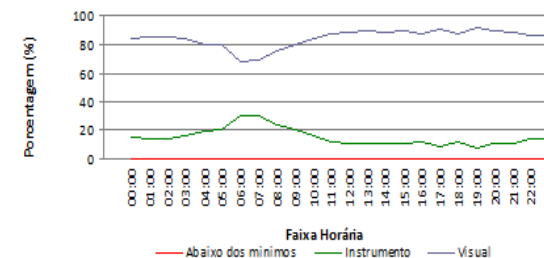
Operacionalidade em porcentagem (Teto 100 ft e visibilidade de 400 m)
